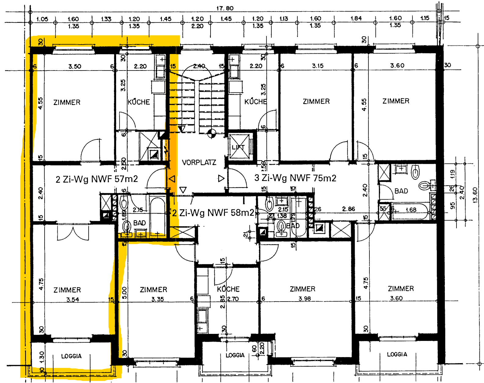
Grundriss 1.-2.-3.-4. OG Mst. :100
