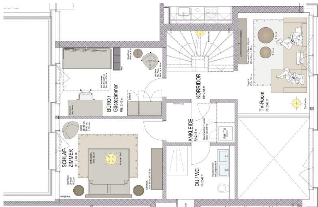
1. OBERGESCHOSS
