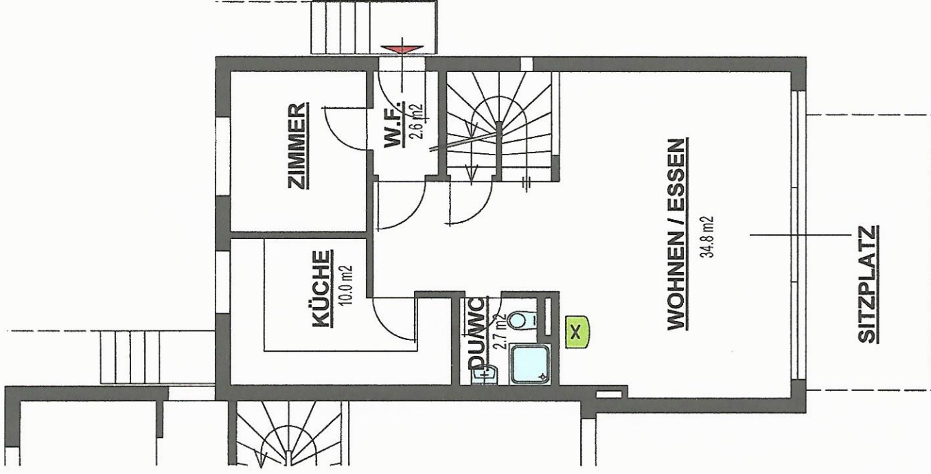
ERDGESCHOSS 1:100
