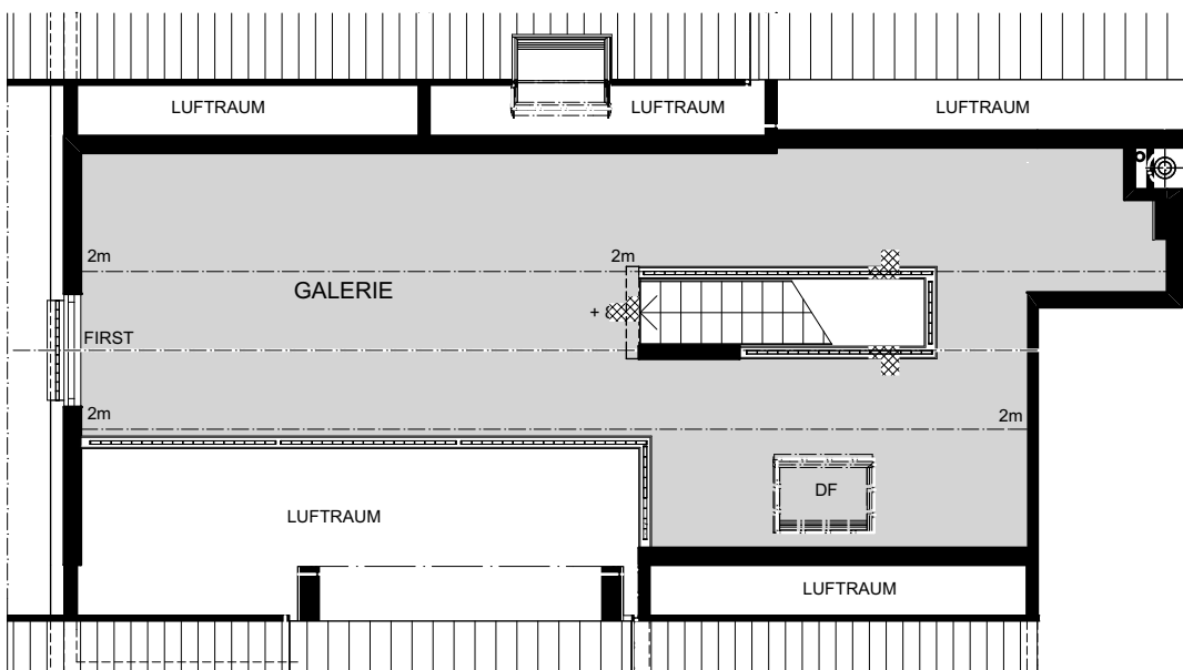
2. DACHGESCHOSS
