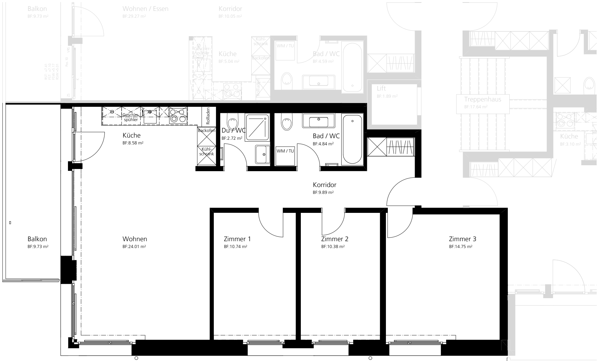
4 1/2 Zimmer Wohnung 85.91m 2
