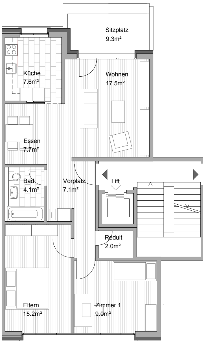
Grundriss MST. 1:100
