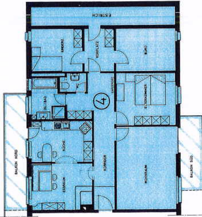
GRUNDRISS MST. 1 : 50
