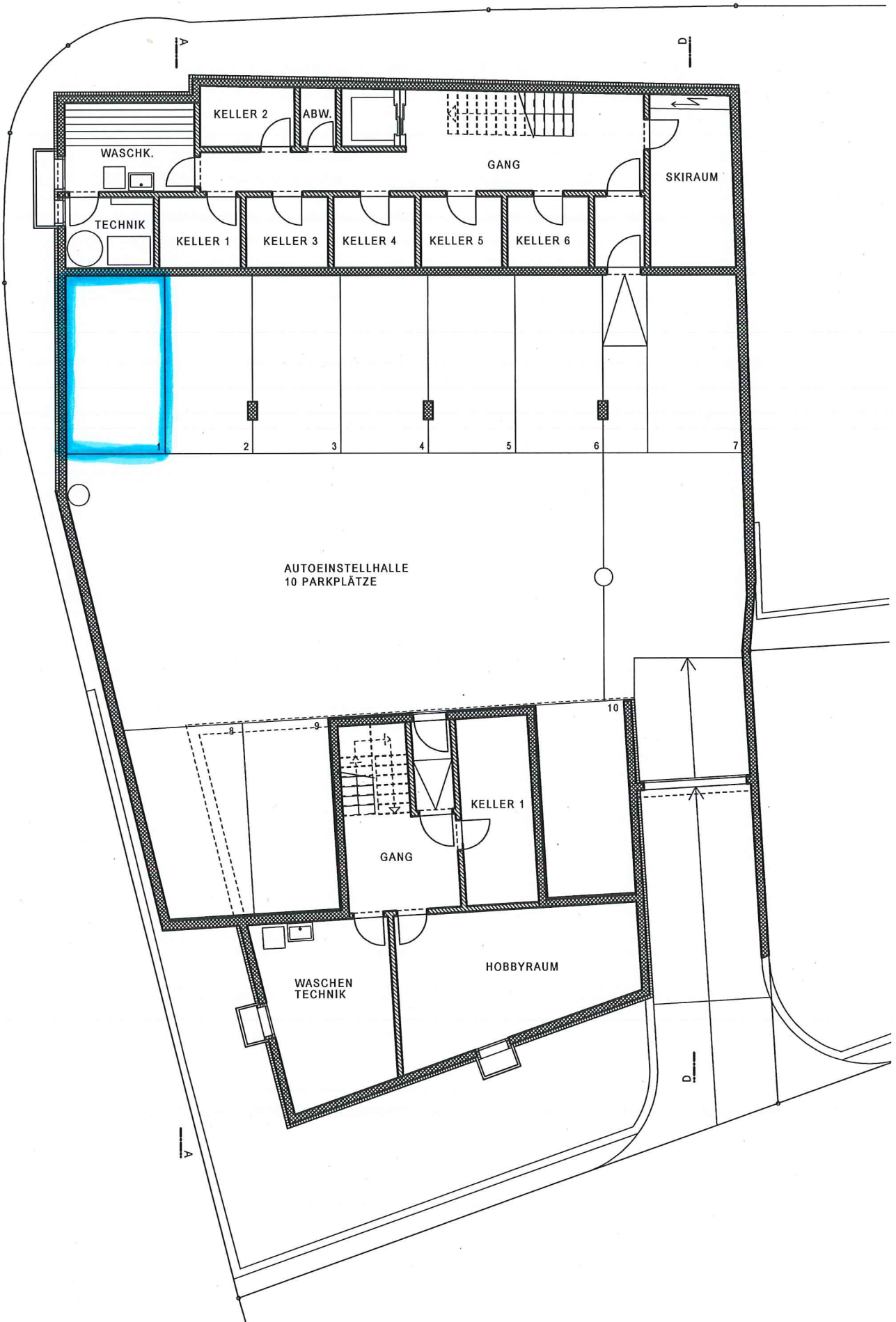
MEHRFAMILIENHAUS DUAL UNTERGESCHOSS
