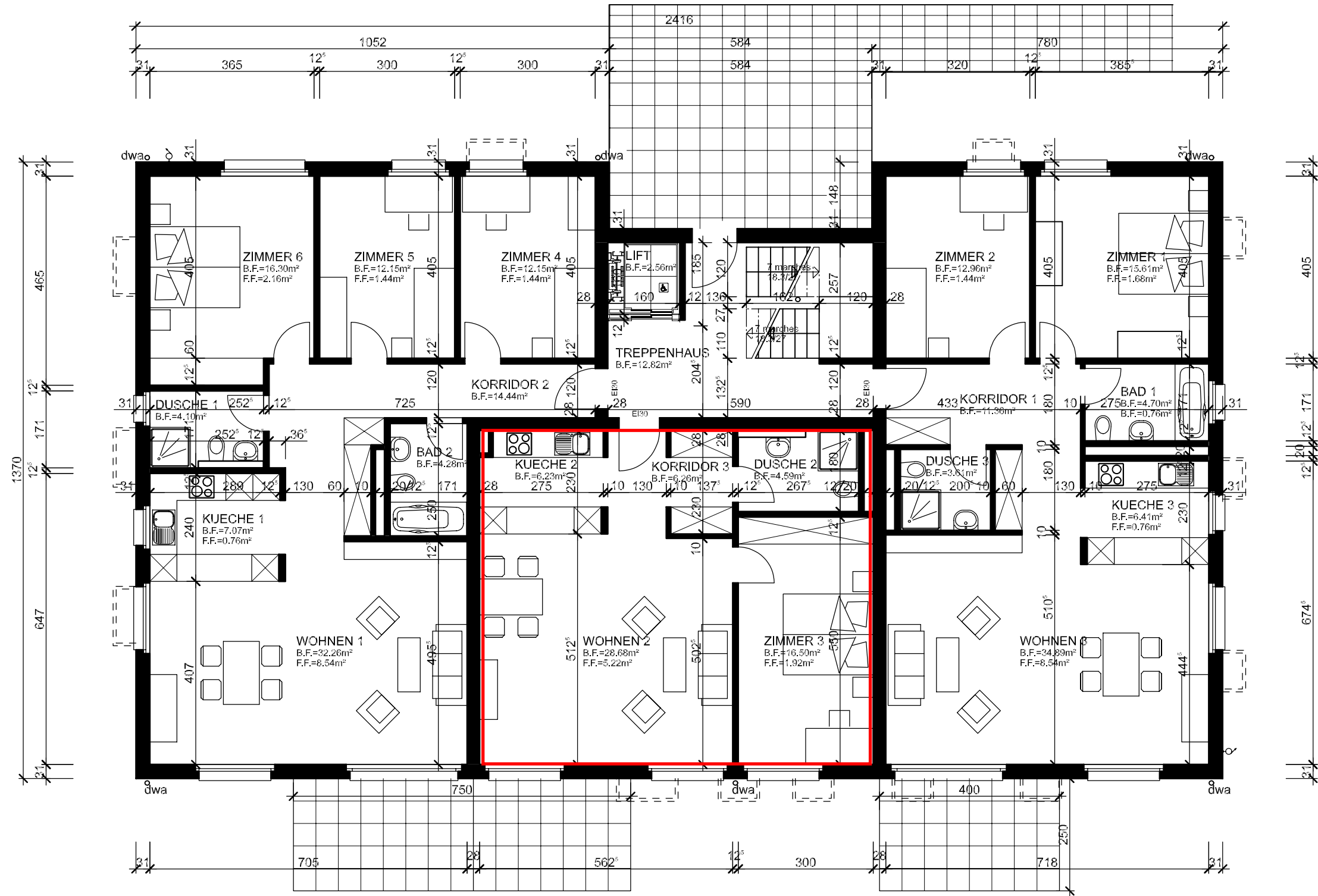
ERDGESCHOSS
