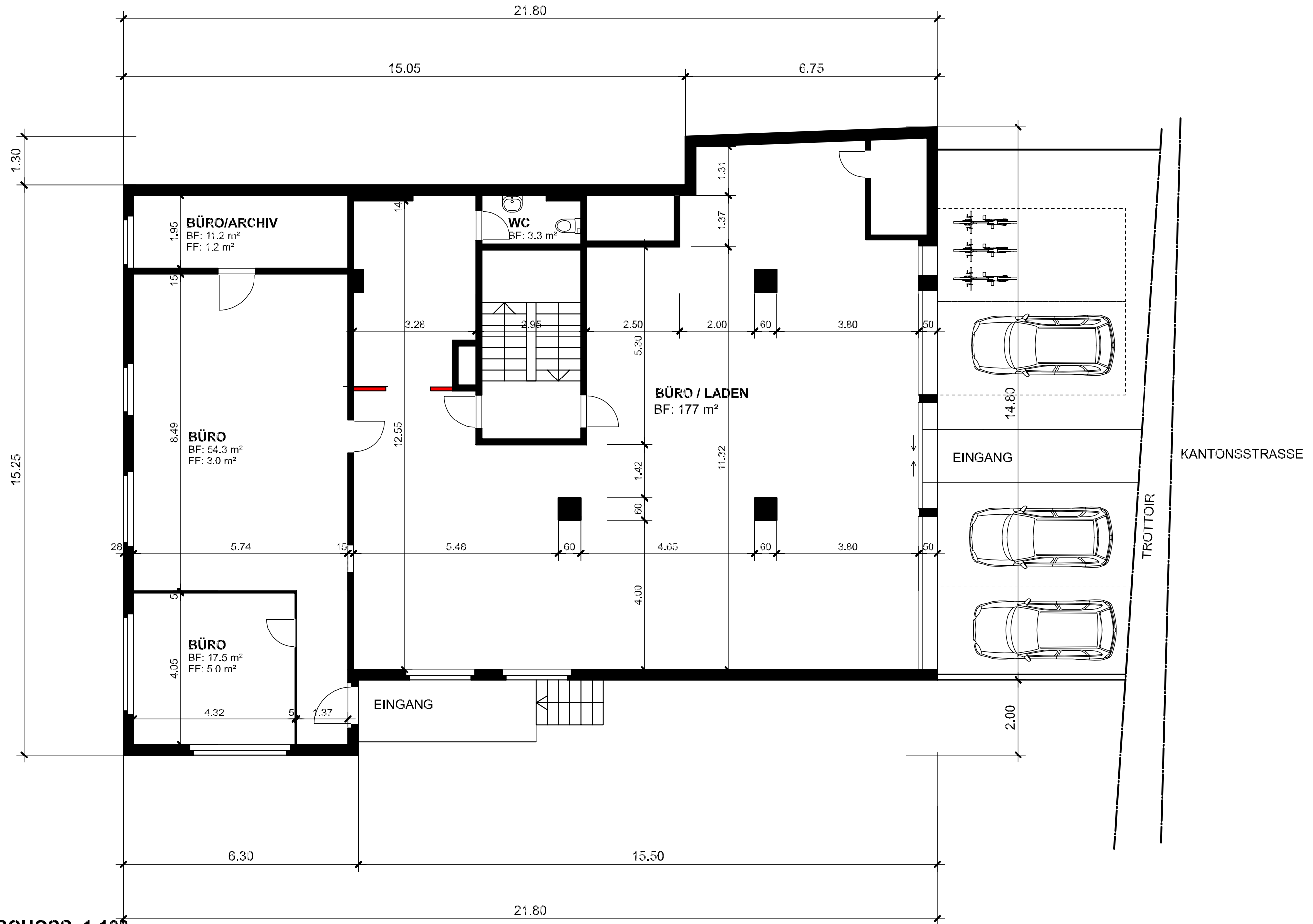
GRUNDRISS ERDGESCHOSS 1:100
